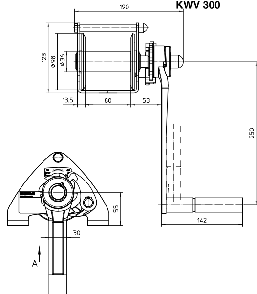
Ansicht A
