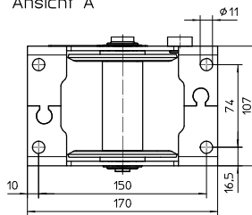
Ansicht A
